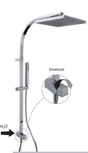
Conjunto ducha anticalcárea CUADRO Ducha fija 250x250 mm. (1.34.138.26). Ducha móvil anticalcárea (006.639.01). Flexo SATIN (91.34.609.15) con toma de agua inferior
