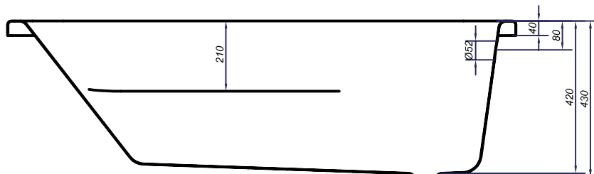
A-A (0,12 : 1)
