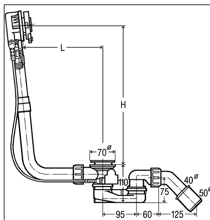
Obr. 3: rozměrový výkres
