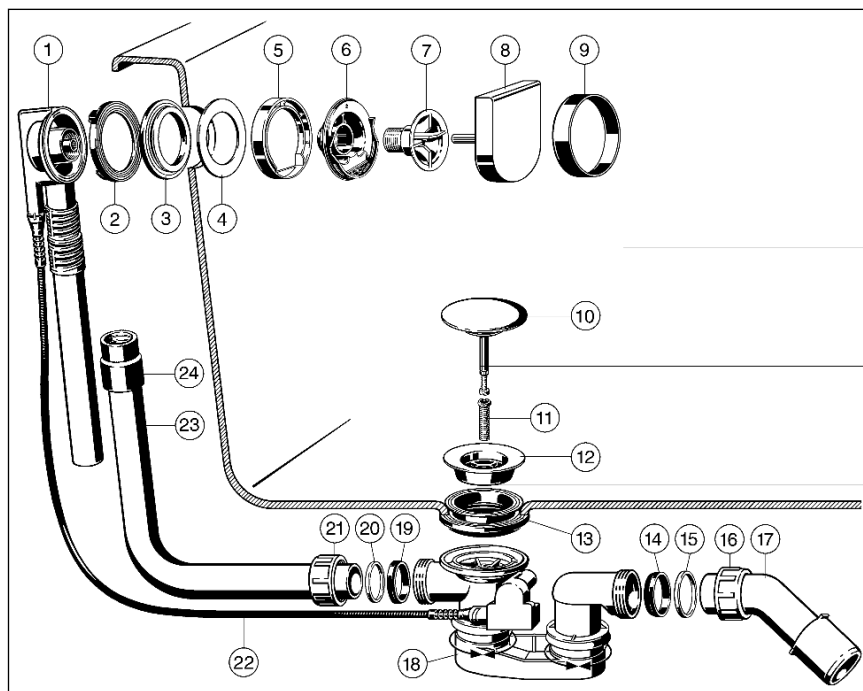
Obr. 1: přehled komponent
