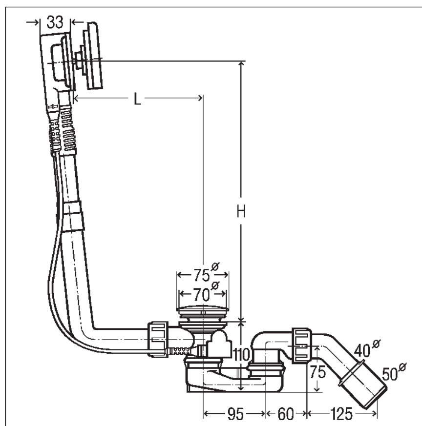
Obr. 2: rozměrový výkres
