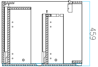
Przekrój A-A
